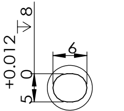
局部视图 D 比例 1.5 : 1
