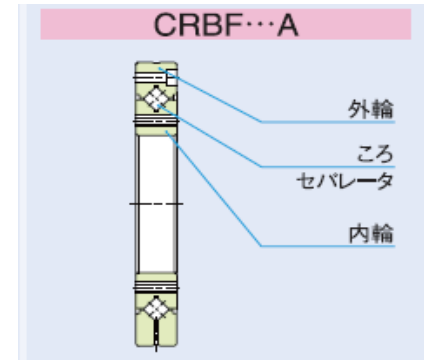
附帶安裝孔的高鋼性交叉滾子軸承
