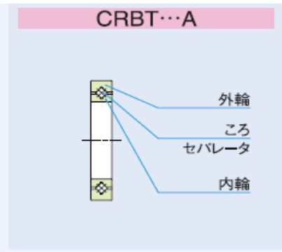
標準型交叉滾子軸承
