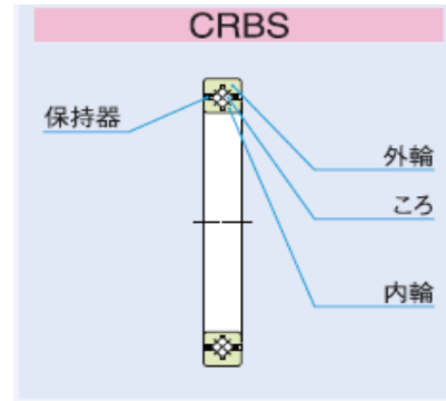
薄型交叉滾子軸承
