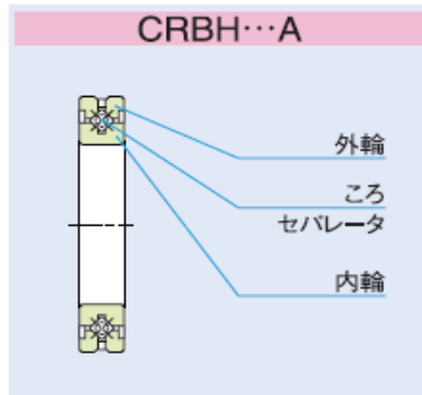
高剛性型交叉滾子軸承
